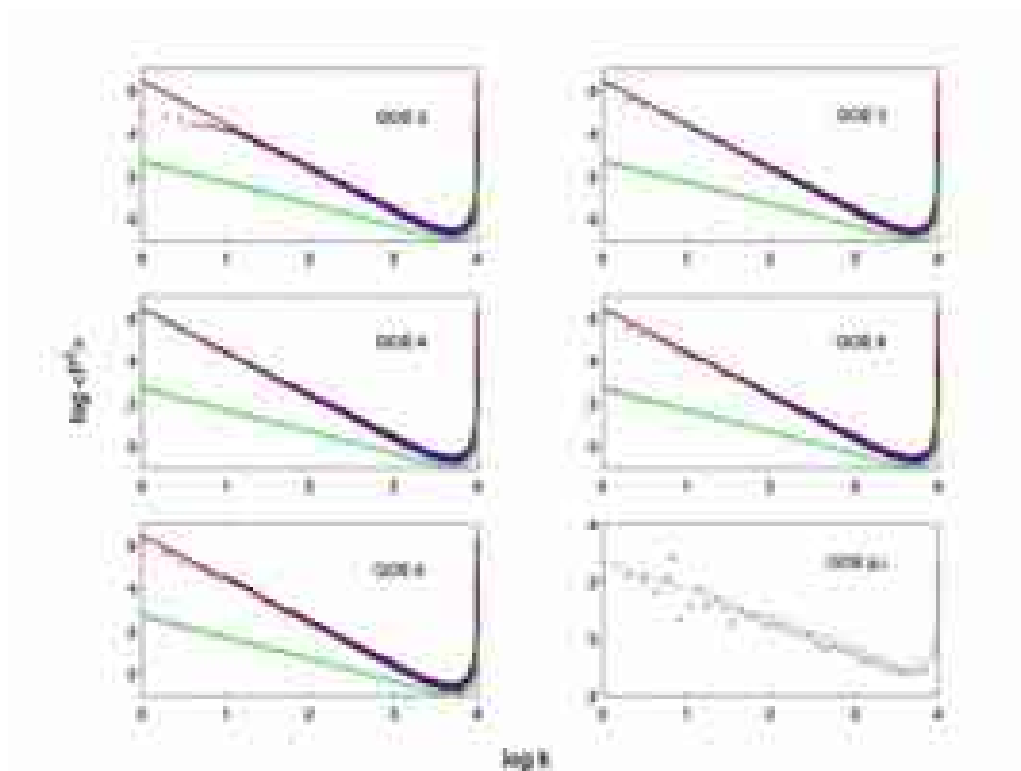
Figura 4.18: Representación del espectro de potencias de los espectros GOE- N y del espectro de partícula independiente tipo GOE junto con las curvas teóricas para GOE (verde) y Poisson (rojo).
