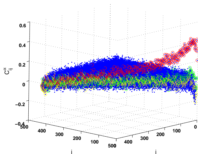
Figura 9.27: Elementos de la matriz de correlación C_{ij}^\alpha correspondiente a la colectividad EGOE(1+2) con \lambda = 0.5 en una representación tridimensional: los índices de fila y columna corresponden a los ejes x e y y el valor del elemento se representa en el eje vertical. Aparecen remarcadas en rojo las correlaciones a primeros vecinos, en verde las correlaciones a segundos vecinos y en amarillo las correlaciones a terceros vecinos.
