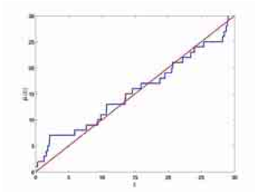
Figura 3.2: Densidad acumulada de un espectro de tipo Poisson reescalado (azul), junto con una recta de pendiente 1 (roja): \mu(\varepsilon) = \varepsilon .
