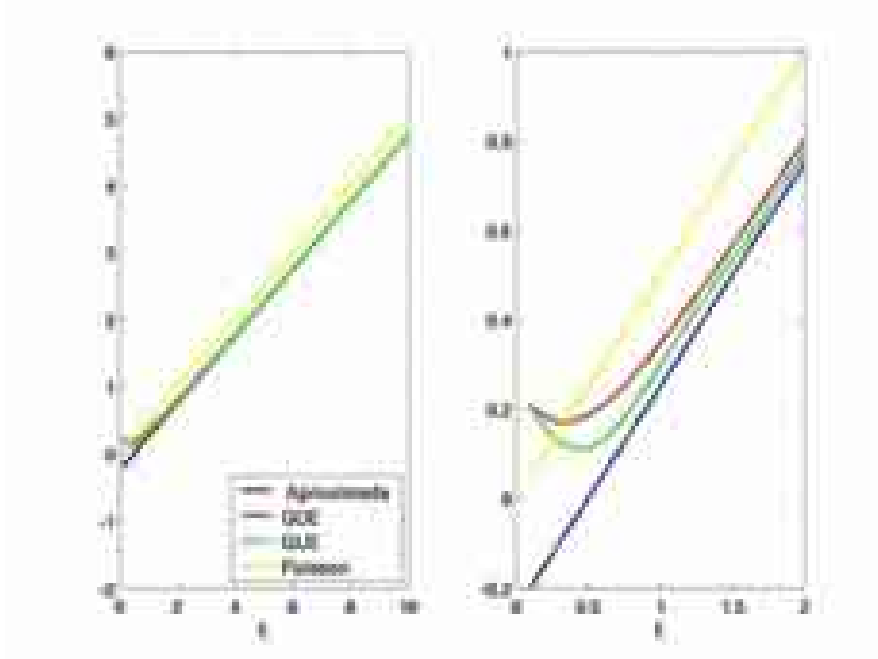
Figura 4.3: En el panel de la izquierda, parte suave de la densidad de estados del sistema de 2 partículas: primera aproximación utilizando sólo \bar{\rho}(E) y curvas exactas para GOE, GUE y Poisson. En el de la derecha una ampliación de la región de energía más baja.
