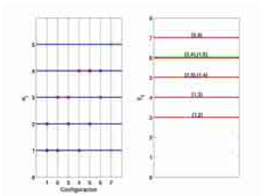
Figura 4.1: Configuraciones posibles de 2 partículas en un espectro de partícula independiente (izquierda) y espectro del sistema de 2 partículas (derecha).
