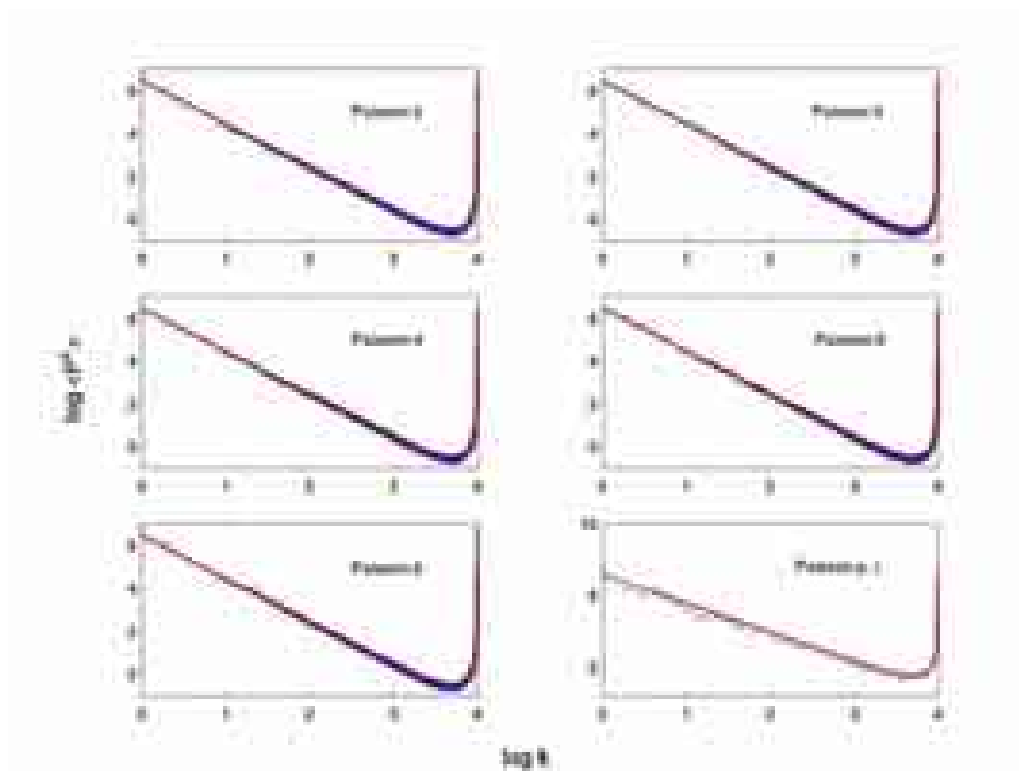
Figura 4.20: Representación del espectro de potencias de los espectros Poisson- N y del espectro de partícula independiente tipo Poisson junto con la curva teórica para Poisson (rojo).
