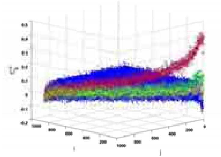
Figura 9.14: Elementos de la matriz de correlación C_{ij}^{\alpha} correspondiente a la colectividad EGOE(2) en una representación tridimensional: los índices de fila y columna corresponden a los ejes x e y y el valor del elemento se representa en el eje vertical. Aparecen remarcadas en rojo las correlaciones a primeros vecinos, en verde las correlaciones a segundos vecinos y en amarillo las correlaciones a terceros vecinos.
